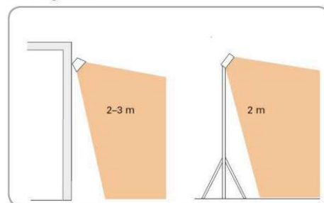
Montagehöhe
